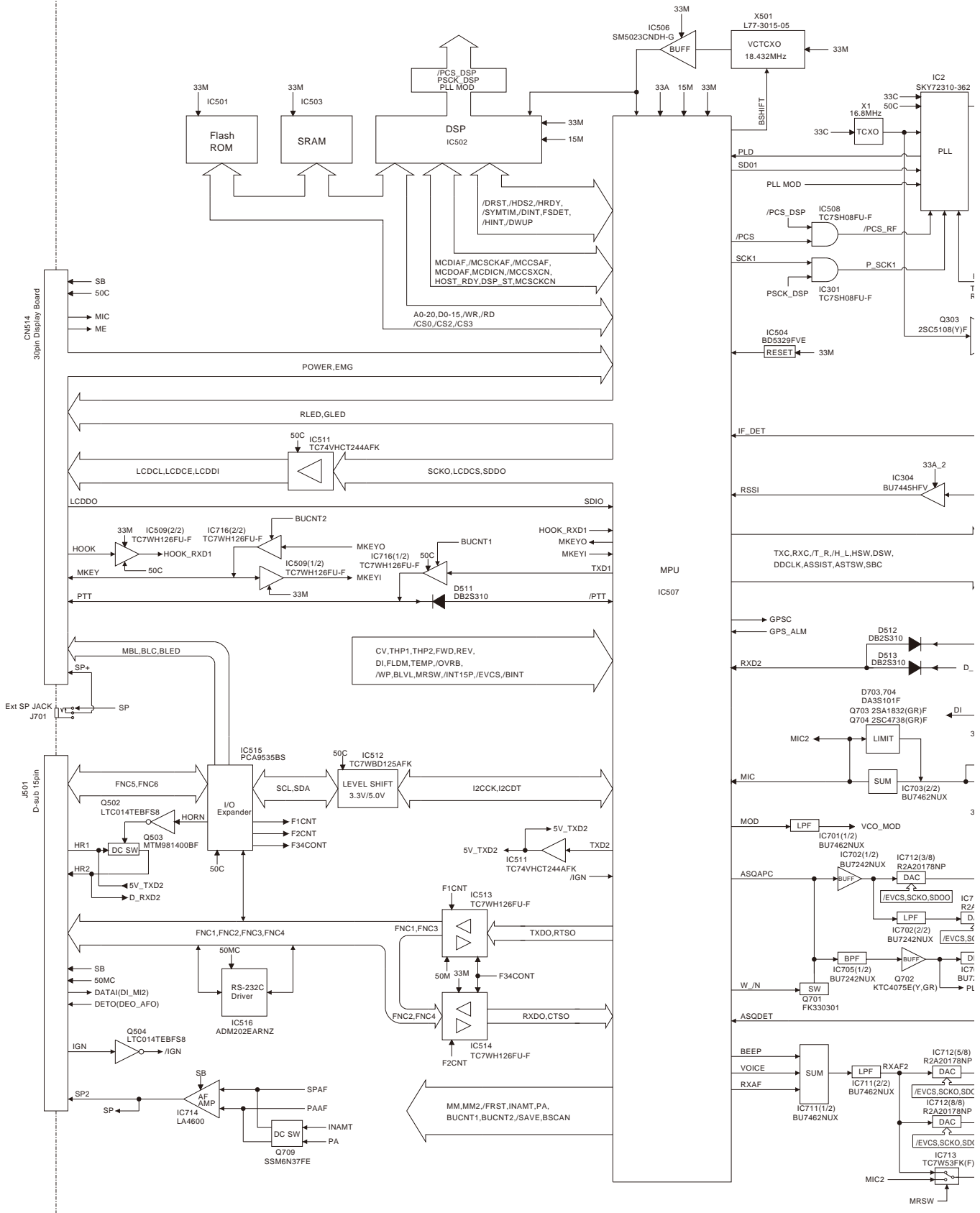
TX-RX UNIT (X57-8230-1X)
